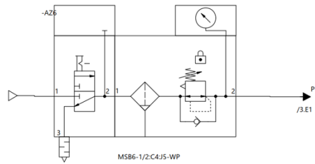
Ausführungsbeispiel Wartungseinheit
