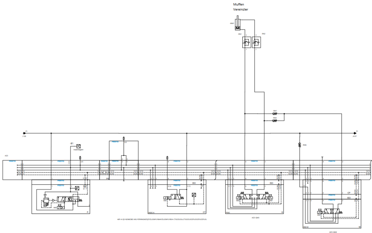
Ausführungsbeispiel Ventilinsel
