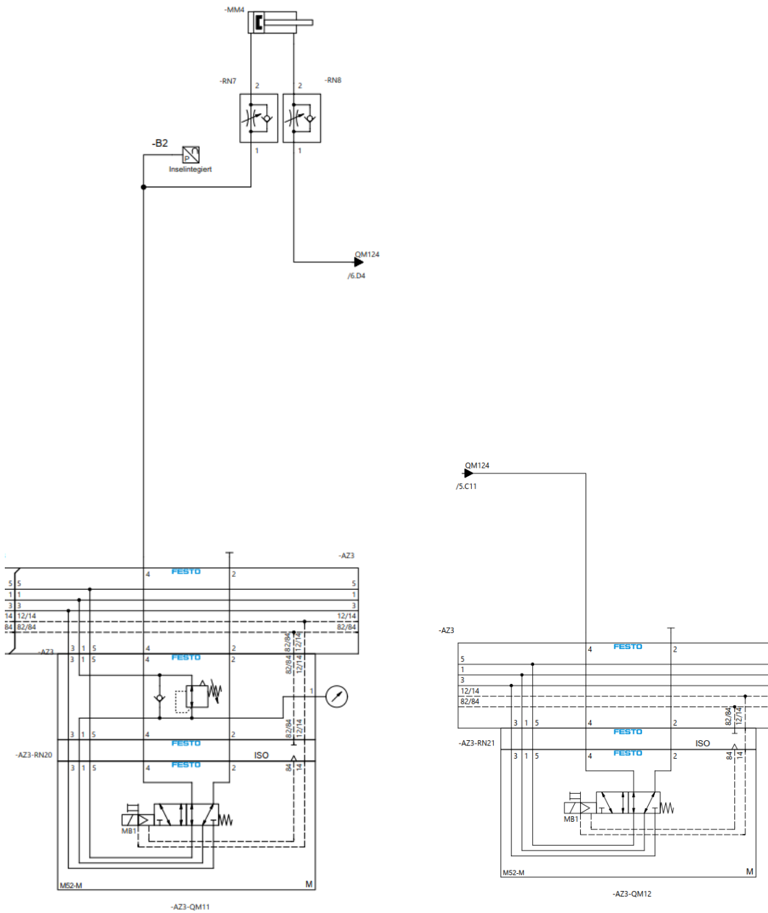
Ausführungsbeispiel für Ventulfunktion mit Druckeinstellung
