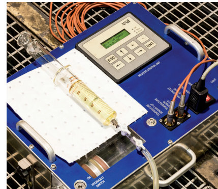
Probenentnahmeggerät
