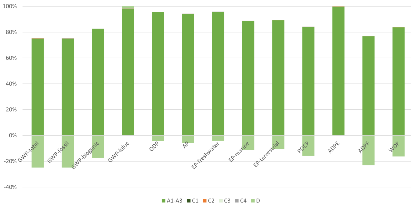
Relative Beiträge der verschiedenen Lebenszyklusphasen von voestalpine walzplattiertes Grobblech (Kupfer)
