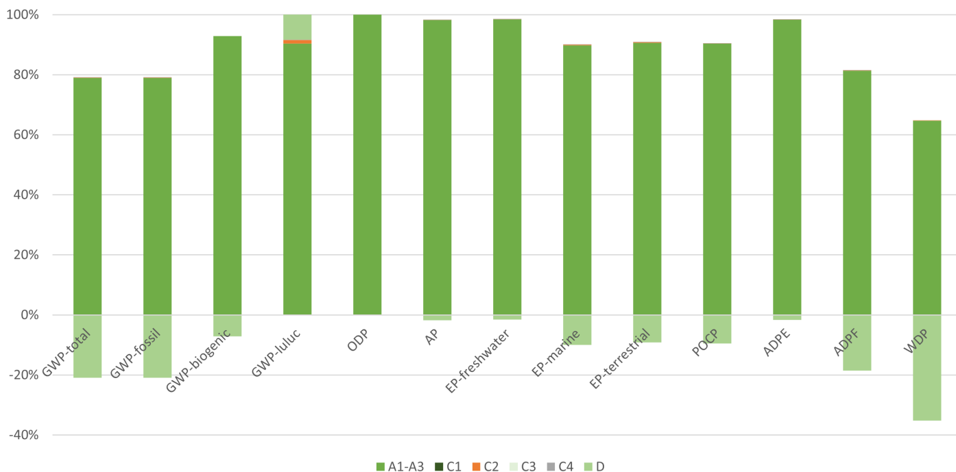
Relative Beiträge der verschiedenen Lebenszyklusphasen von voestalpine walzplattiertes Grobblech (UNS N08825 / 2.4858)
