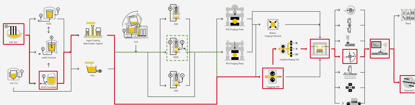
Processus de production du A204: — = A204, - - - = A224 (pour la signification des acronymes, se référer au lexique p38)
