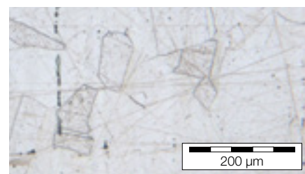
microstructure 1.4435 conventionnel
