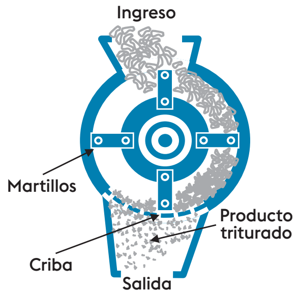
Diagrama de molienda
