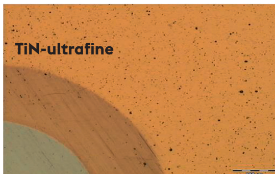
Oberfläche mit Kalottenschliff einer Standard TiN (oben) und einer TiN-ultrafine.
